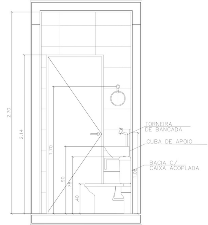
CORTE BB FUNCIONÁRIOS
