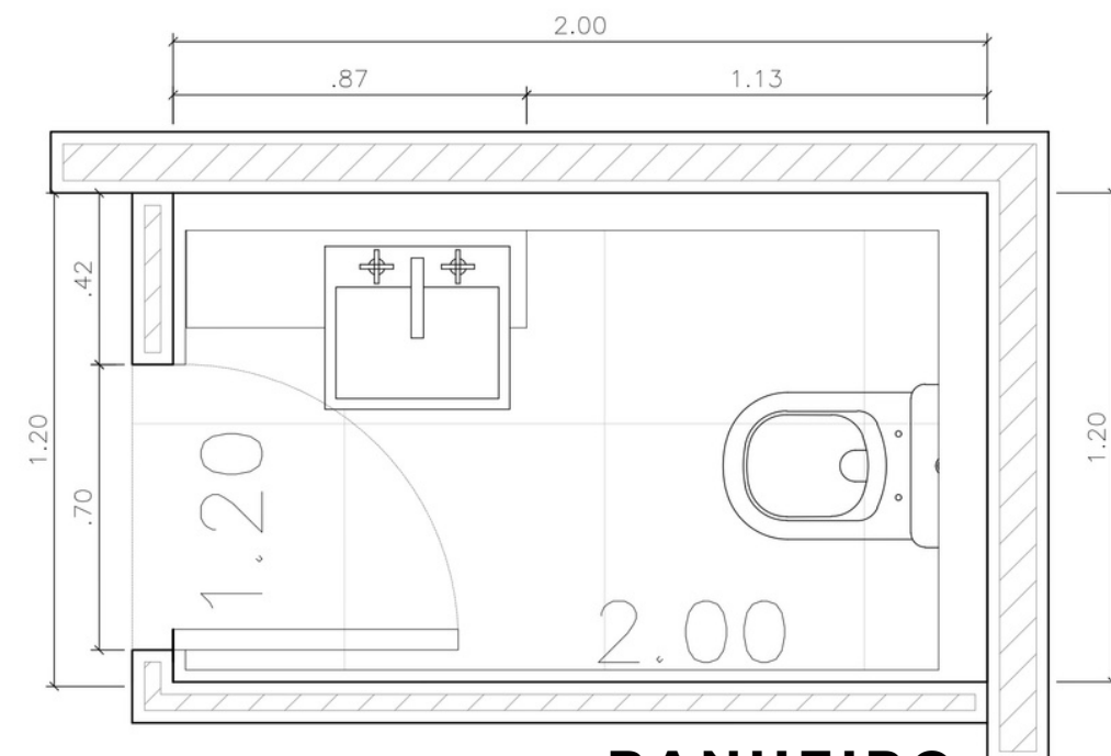
BANHEIRO SALÃO.
