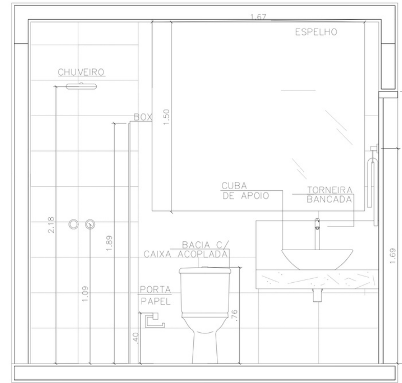
CORTE AA FUNCIONÁRIOS
