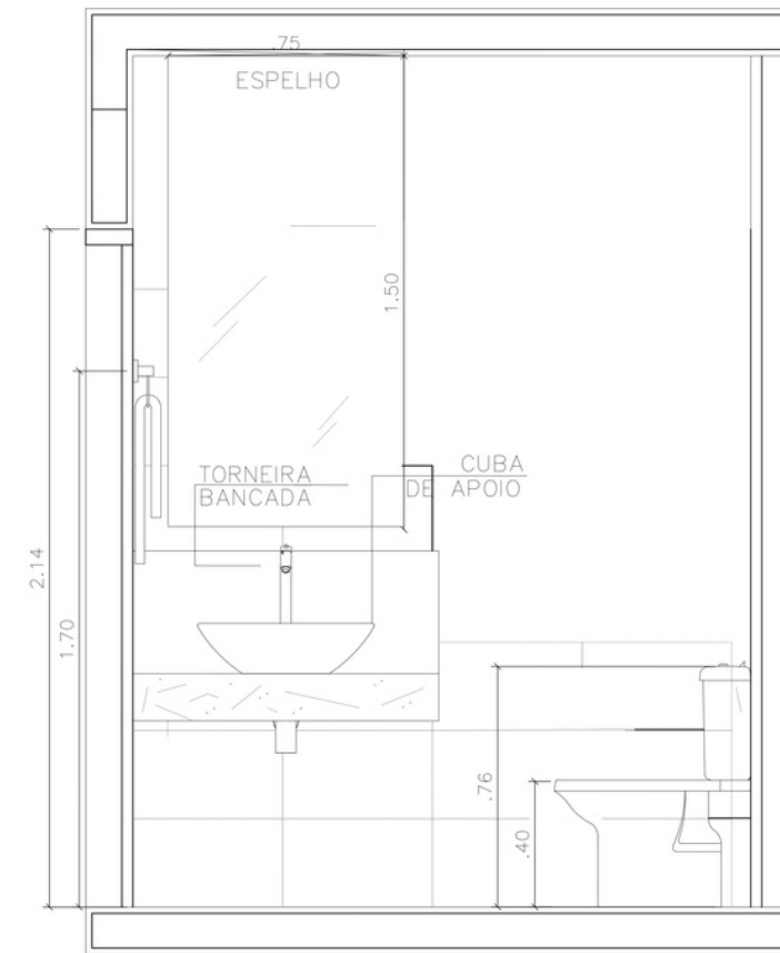
CORTE AA SALÃO.
